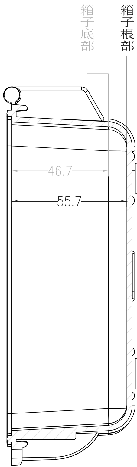
剖面 B-B
